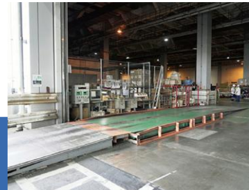
20フィートピットスケール ひょう量：20t
